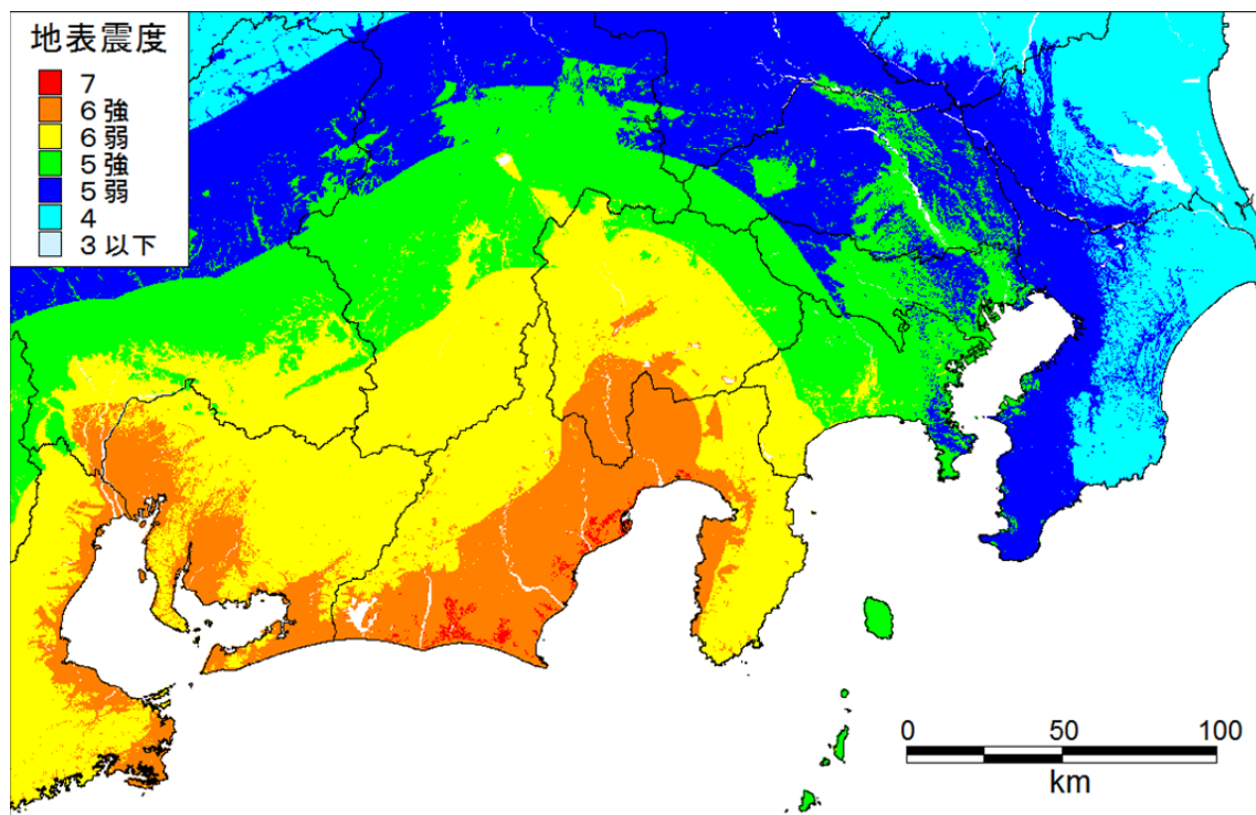
経験式 地表震度_関東-中部
