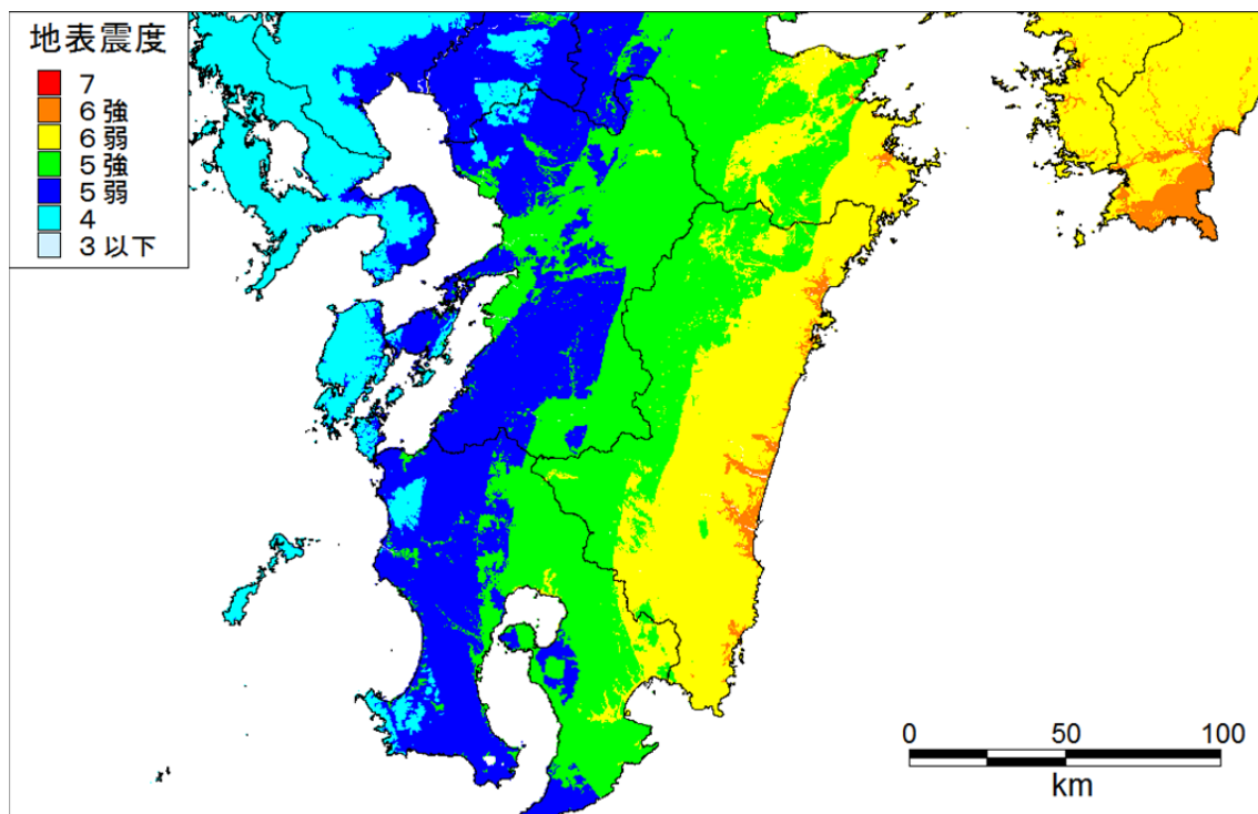
経験式 地表震度_九州
