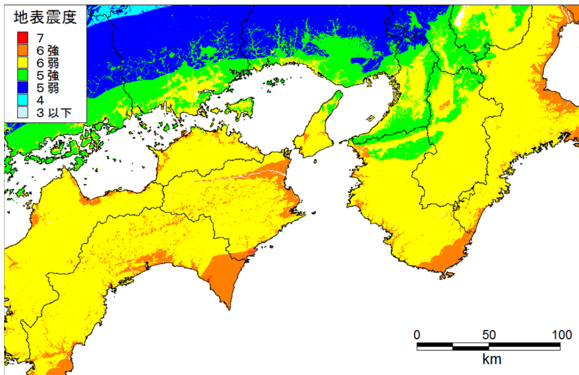
経験式 地表震度_近畿-四国
